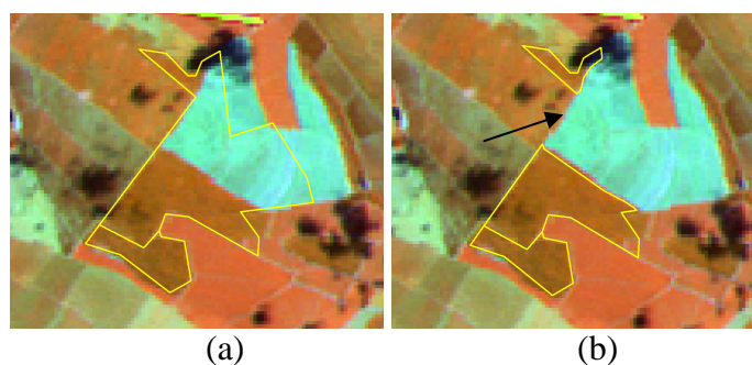
Figura 3. Exemplo de identificação de desmate nos polígonos de RVN. Imagem TM, composição R(4) G(5) B(3), de 29/04/2009. Em: a) polígono original de RVN, em amarelo, sobreposto na imagem TM; e b) polígono editado de RVN, em amarelo.
