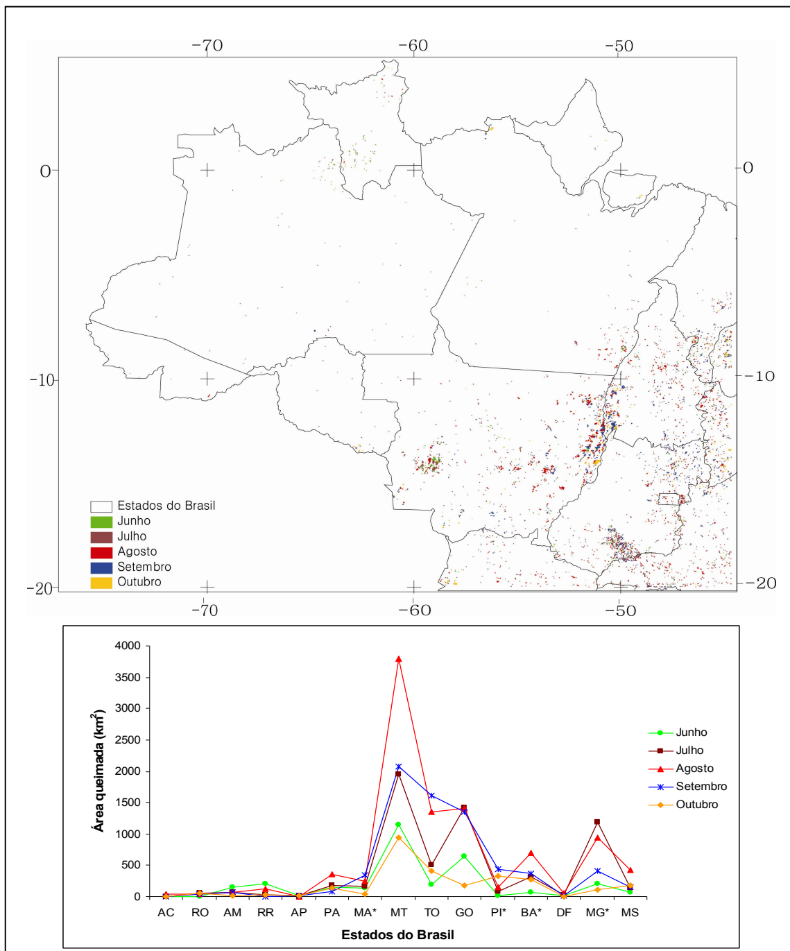
Figura 3. Área queimada na Amazónia brasileira no ano 2000, entre Junho e Outubro.
