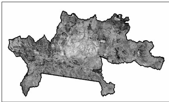
Figura 6: Imagem-fração sombra do MNAFTO.
