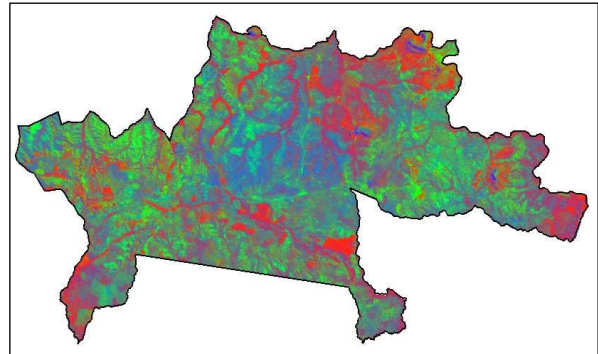
Figura 7: Composição colorida de imagens-fração (Vermelho-vegetação; Verde-solo e Azul-sombra) do MNAFTO.
