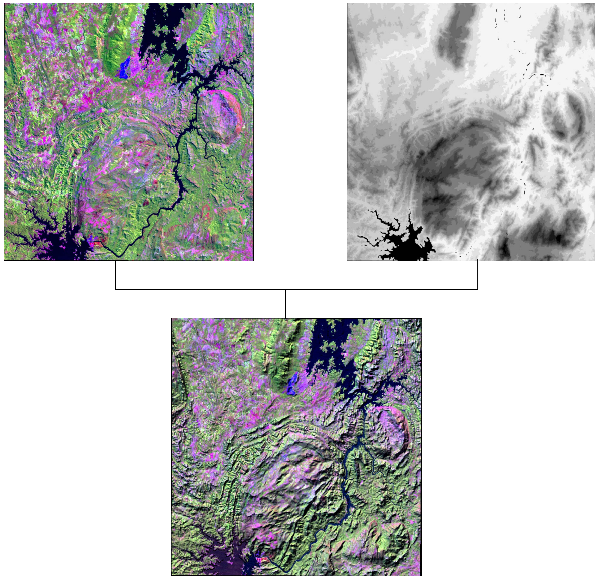
Figura 2: Imagem Landsat 7 ETM+ 2003 bandas 543 RGB (acima à esquerda); Grid SRTM 90 (acima à direita); Integração Imagem x MDT – Sombreamento de relevo (abaixo ao centro)
