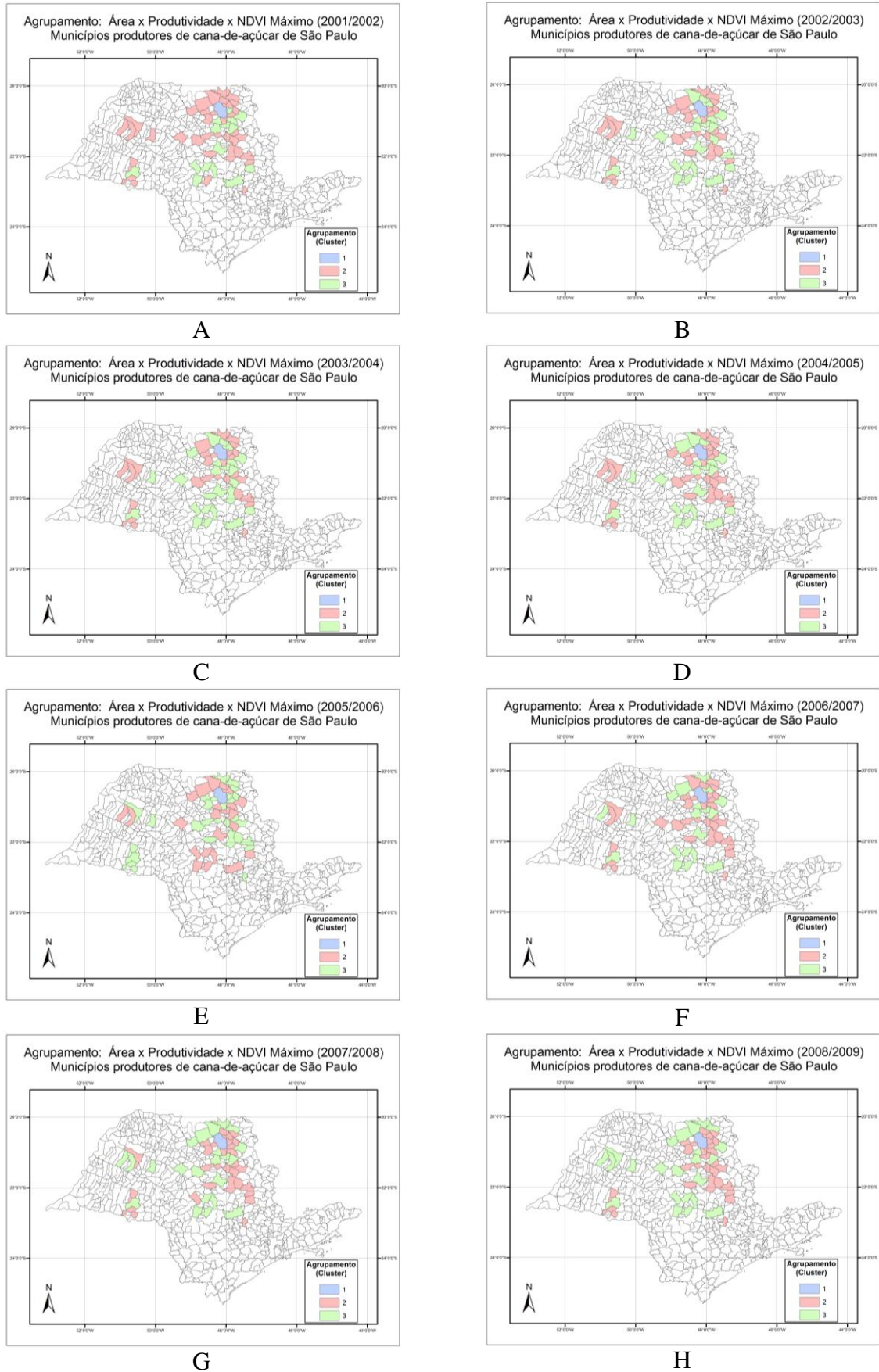
Figura 4. Agrupamento das variáveis, área plantada, produtividade e NDVI máximo para os 50 municípios produtores de cana-de-açúcar nas safras 2001/2002 a 2008/2009.
