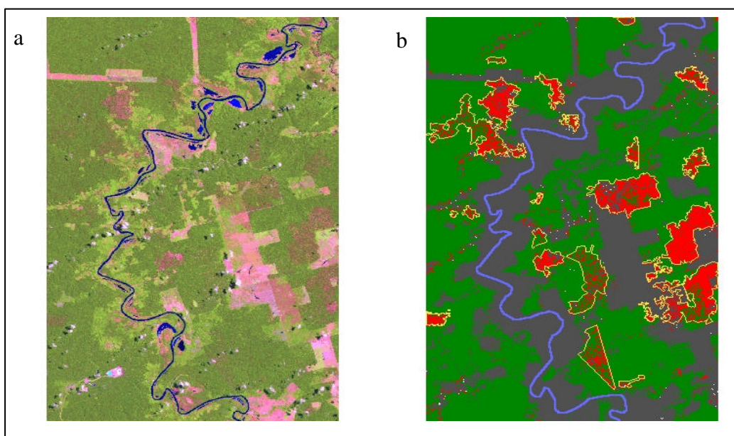
Figura. 1. a) Imagem TM-Landsat (data), bandas 3 (R), 4 (G) e 5 (B), Baixo Rio Capim, PA e b) imagem classificada resultante do uso do algoritmo de Máxima Verossimilhança, indicando, em vermelho, as áreas afetadas pelo corte seletivo; em verde, as áreas de florestas; e, em preto, as áreas não florestadas. Os polígonos envolventes utilizados no cálculo da área associada à exploração madeireira estão representados em amarelo.
