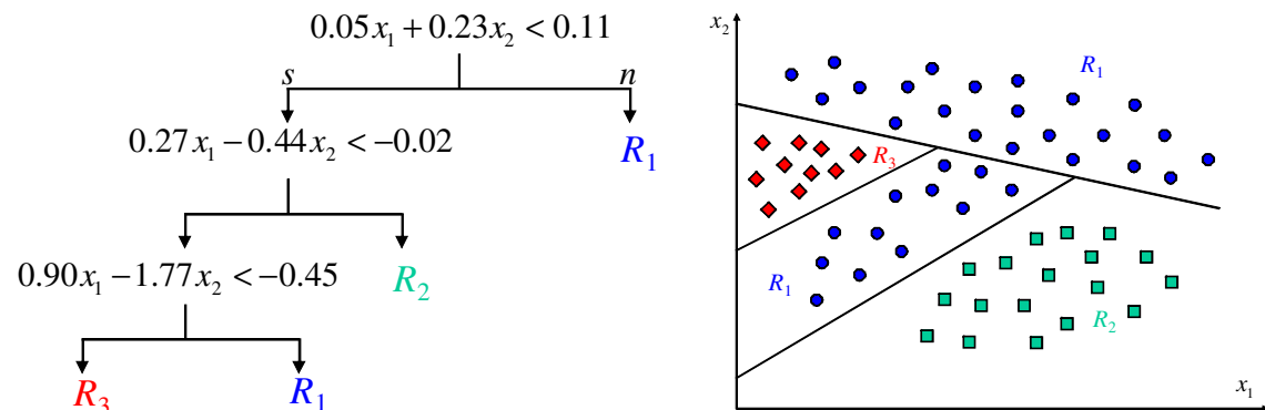
Figura 2. Exemplo de árvore de decisão oblíqua. Adaptado de Duda et al. (2001)
