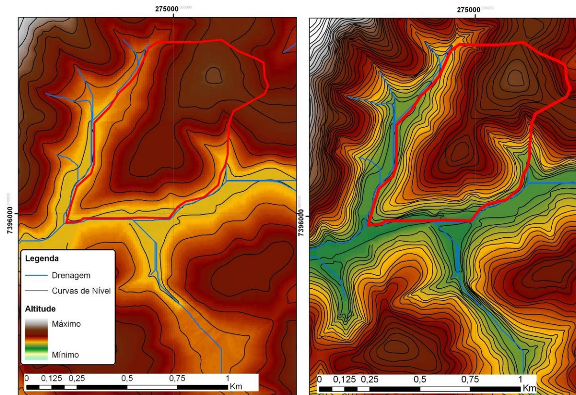
Figura 2. Diferença entre as curvas de nível e o modelo digital de terreno nas escalas 1:50.000 (à esquerda) e 1:10.000 (à direita), e localização da feição do terreno analisada (contorno em vermelho).
