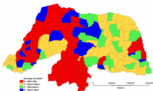
Figura 2 – Mapa de espalhamento de Moran para IDHM do RN. Fonte dos dados: Atlas de Desenvolvimento Humano Municipal, 2000.
