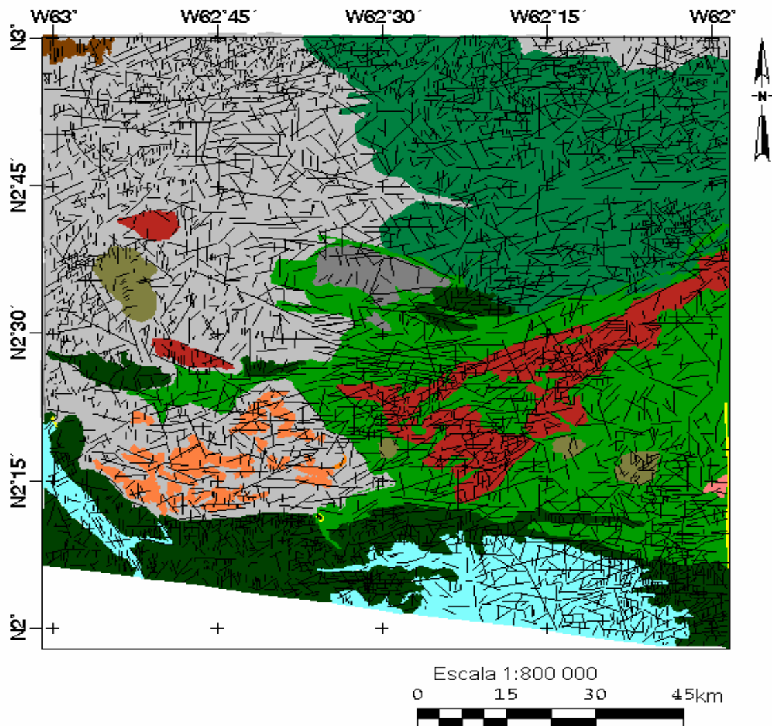
Figura 2. Mapa geológico e estrutural final da região do Rio Mucajaí.
