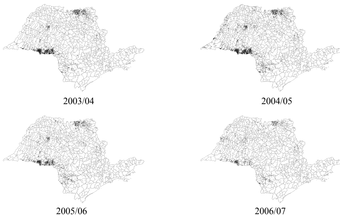
Figura 2. Áreas plantadas com soja selecionadas pela máscara, nas safras 2003/04 a 2006/07.
