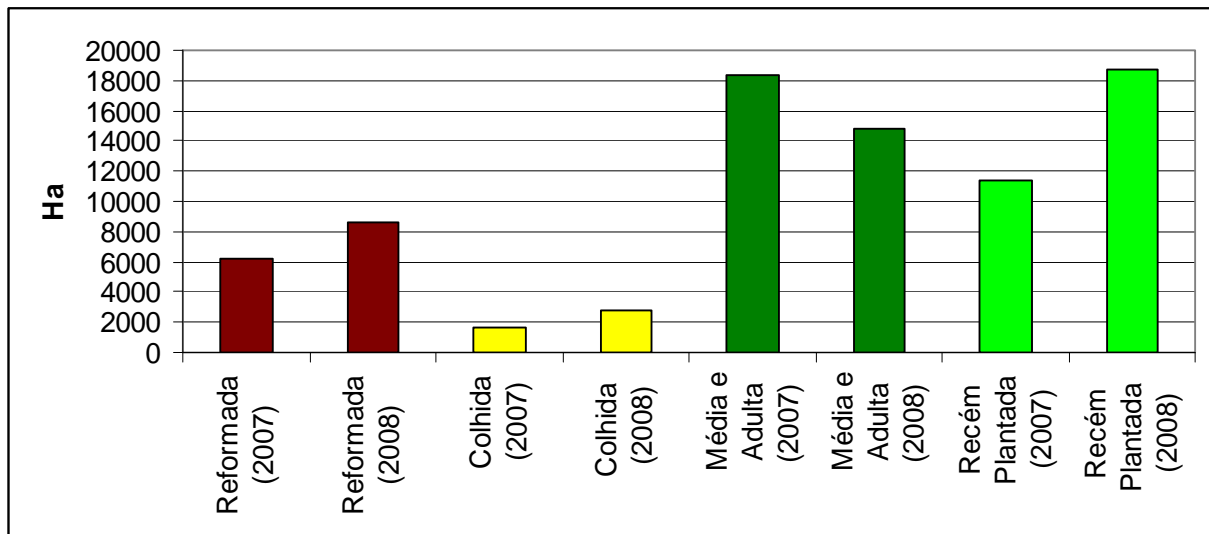
Figura 8. Comparativo das categorias das áreas ocupadas com cana-de-açúcar no município de Campo Florido-MG para o mês de agosto de 2007 e 2008.
