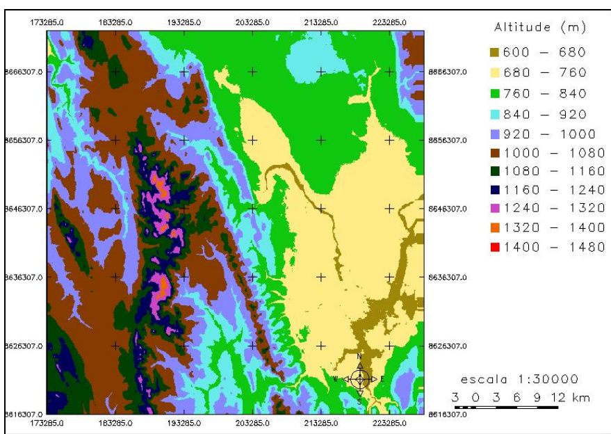
Figura 4 – Mapa hipsométrico da Folha Seabra, BA.
