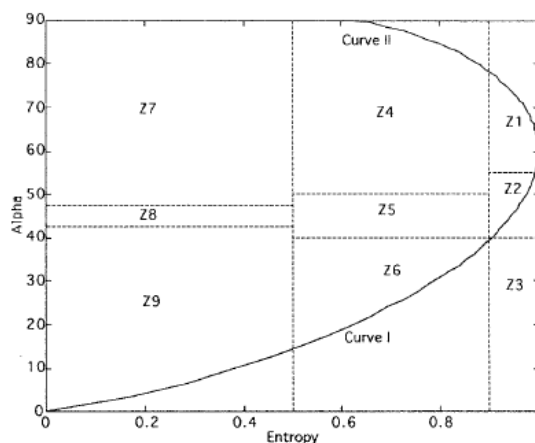
Figura 1. Plano com a entropia (H) e alpha ( \alpha ).
