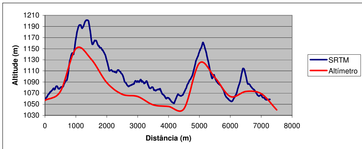
Figura 8. Comparativo entre os perfis altitudinais da trilha do rio Bonito obtidos em campo com altímetro e com dados do SRTM.
