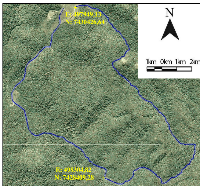
Figura 2. Mosaico das fotografias aéreas ortoretificadas do PESH Núcleo Cunha, integradas no SPRING, com o traçado da Trilha do Rio Bonito obtido pela interpretação do mosaico.
