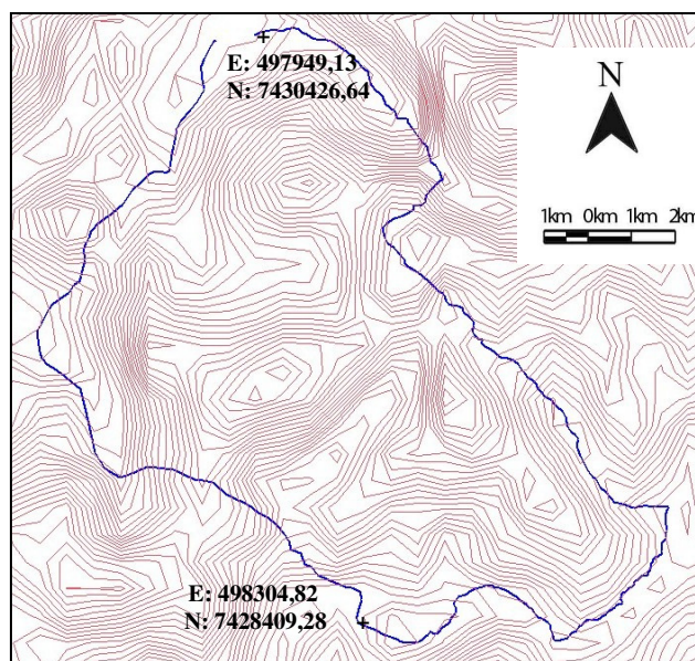
Figura 4. Curvas de nível a cada 10 metros derivadas a partir de Modelo Numérico do Terreno derivado do SRTM, sobrepostas pelo traçado da Trilha do Rio Bonito obtido a partir da interpretação das fotografias aéreas ortorretificadas.
