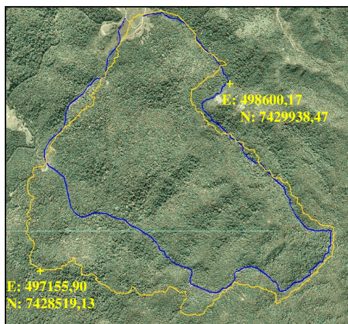
Figura 6. Traçados da Trilha das Cachoeiras sobre o mosaico ortorretificado; em azul, o traçado obtido com informações interpretadas diretamente sobre o mosaico e em amarelo, traçado obtido usando bússola e trena.
