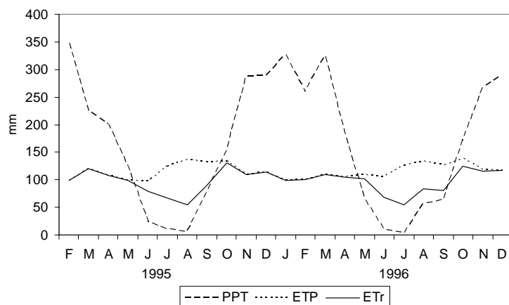
Figura 4 – Balanço hídrico da bacia do Ji-Paraná, obtido pelo modelo
