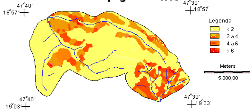
FIG.7 - Fator Topográfico -1998
