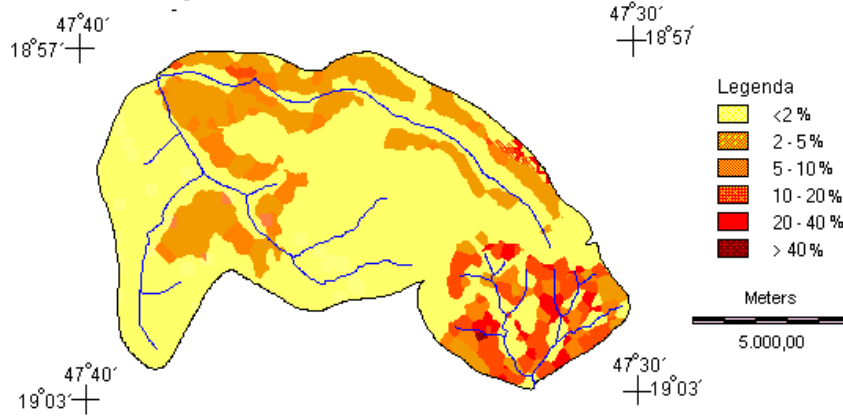
FIG.5-Mapa de Declividade-1998
