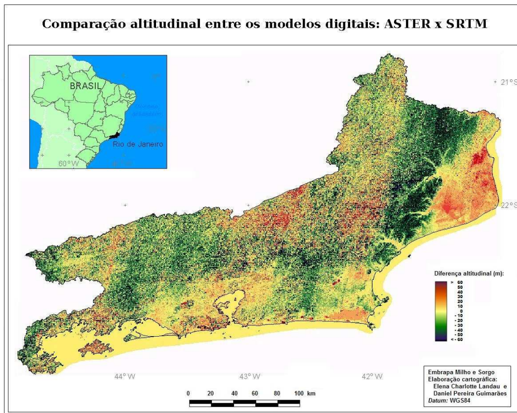
Figura 2. Imagem resultante da subtração dos MDEs extraídos dos sensores ASTER e SRTM para o Estado do Rio de Janeiro, Brasil.
