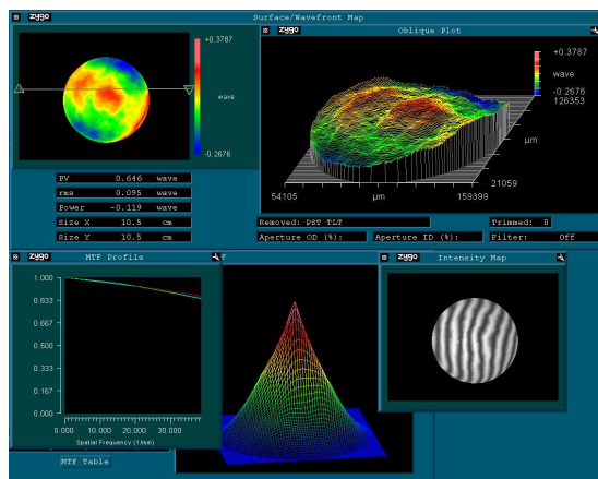
Figura 8 – Interferograma e curvas de MTF do sistema óptico MUX, no field central, capturada com o interferômetro Zygo. FONTE: Opto Eletrônica S.A.
